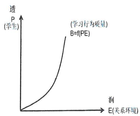
图3 行为质量、关系环境函数变化关系
